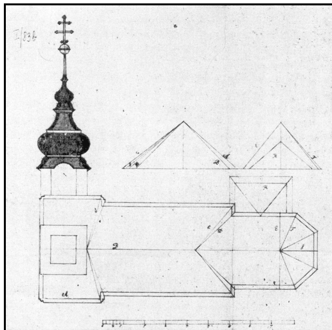
Ifj. Zwenger József templombővítési rajza 1830-ból
