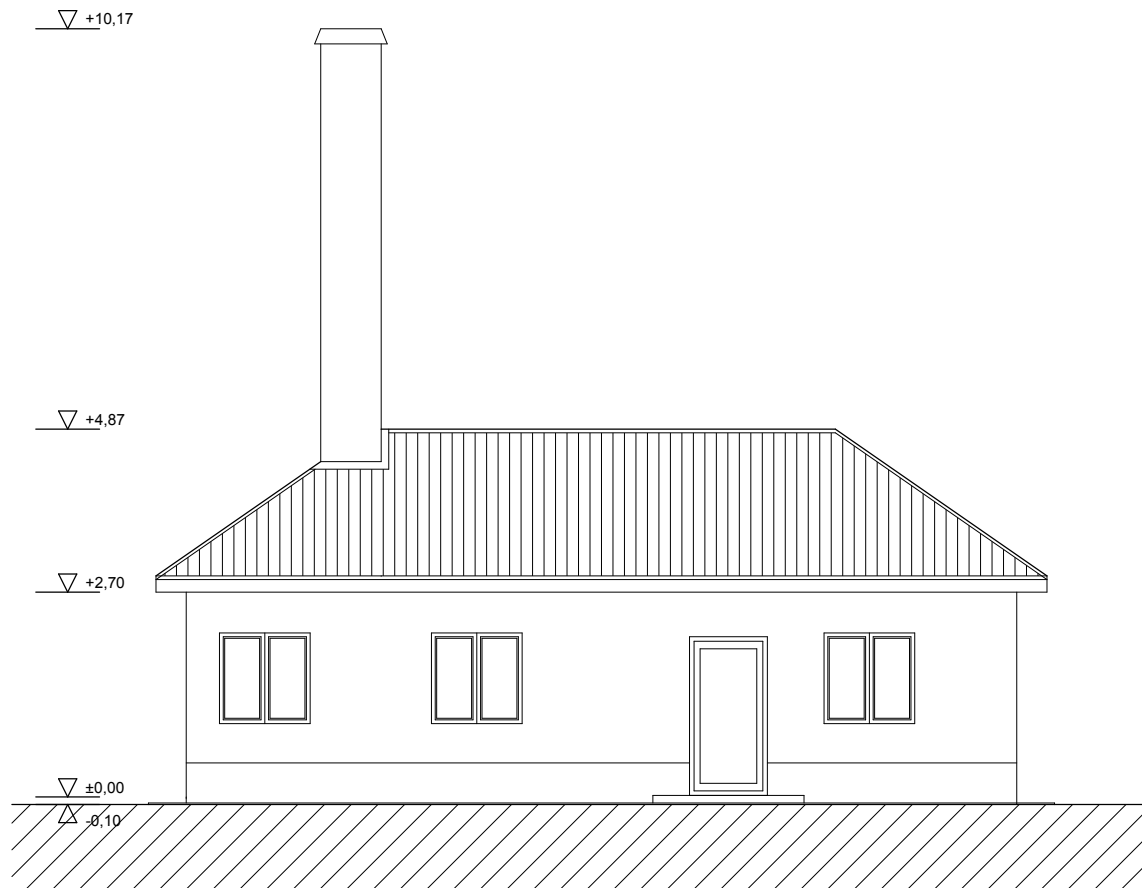
Északkeleti homlokzat
