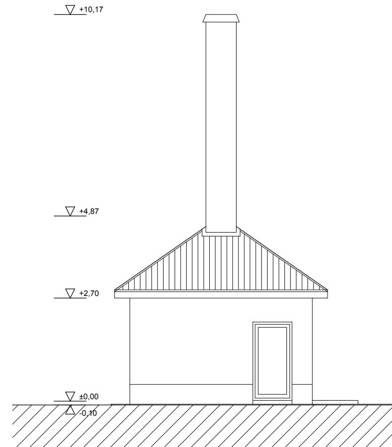
Délkeleti homlokzat
